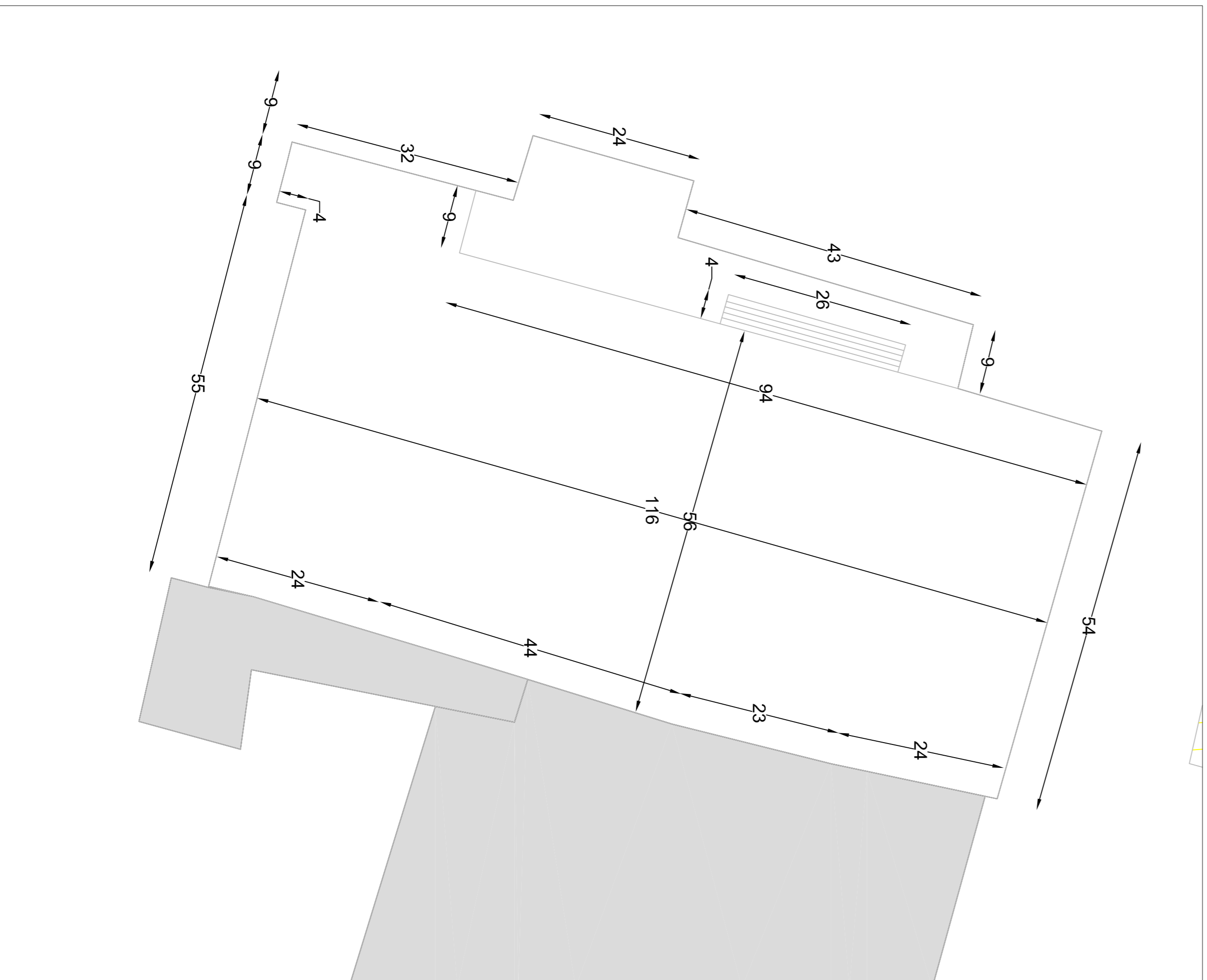
RILIEVO STATO DI FATTO scala 1:500
